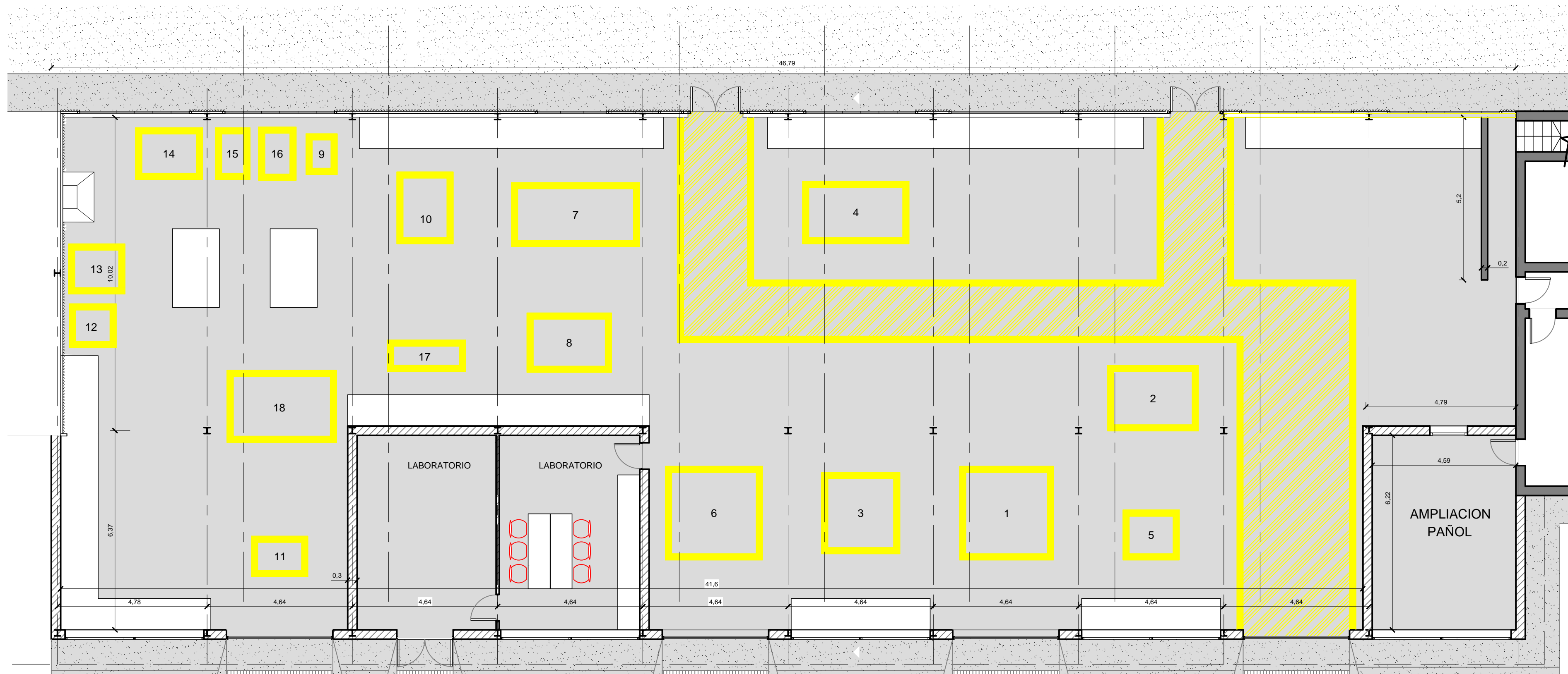
DISTRIBUCION DE MAQUINARIA Y PASILLO PEATONAL ESC. 1/100
