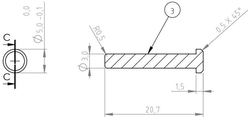
SECCIÓN C-C ESCALA 2 : 1
