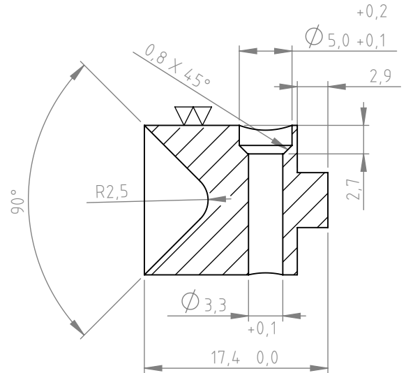
SECCIÓN A-A ESCALA 2 : 1
