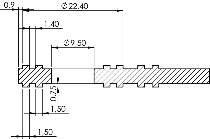
SECCIÓN B-B ESCALA 2 : 1
