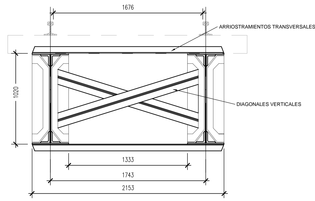
CORTE 1-1 ESCALA 1:20 Medidas en mm
