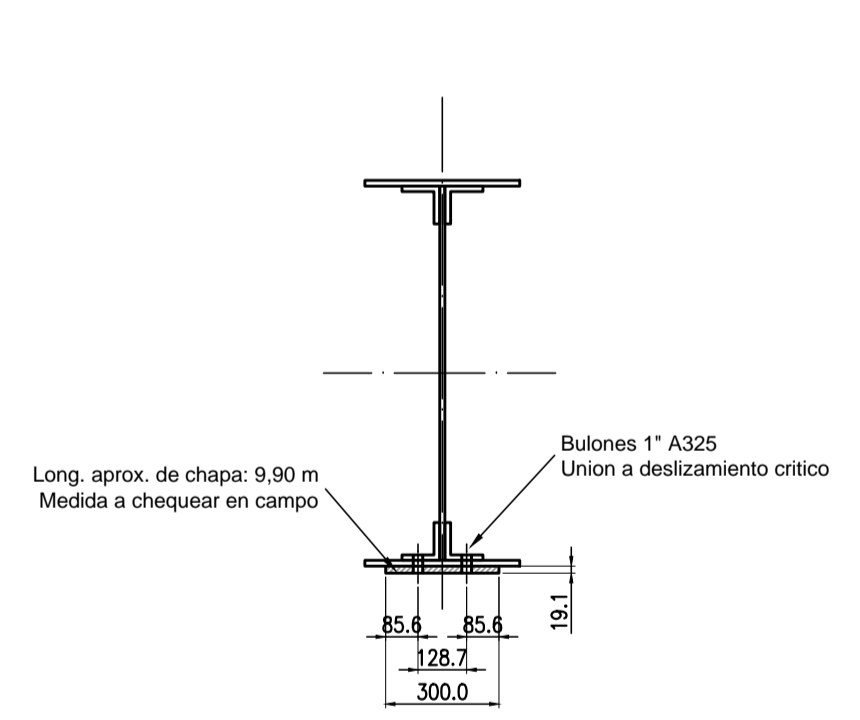
REFUERZO ALA INFERIOR ESCALA 1:20 Medidas en mm
