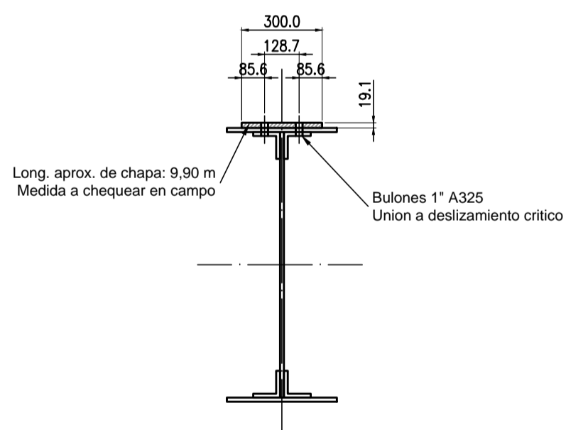
REFUERZO ALA SUPERIOR ESCALA 1:20 Medidas en mm
