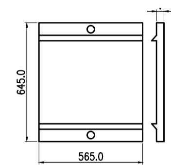
PLACA DE APOYO ESCALA 1:20 Medidas en mm
