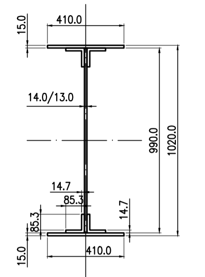
SECCION VIGA PRINCIPAL ESCALA 1:20 Medidas en mm
