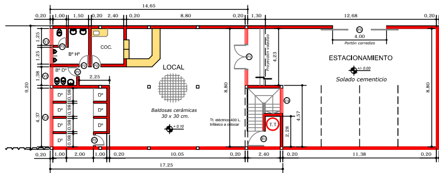
PLANTA BAJA Altura interior de los locales a construir 3.50 m.
