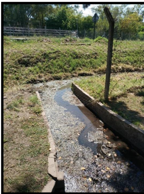
Ilustración 3. Desagüe de calle/boca tormenta que finaliza en zanja de vía
