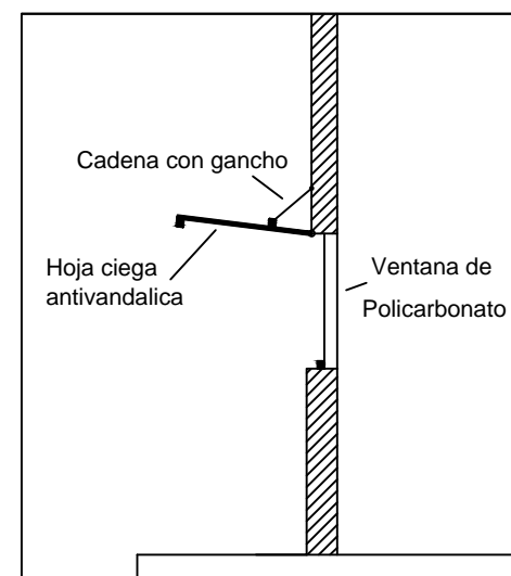
DETALLE ABERTURA
