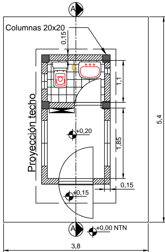
PLANTA +0.20
