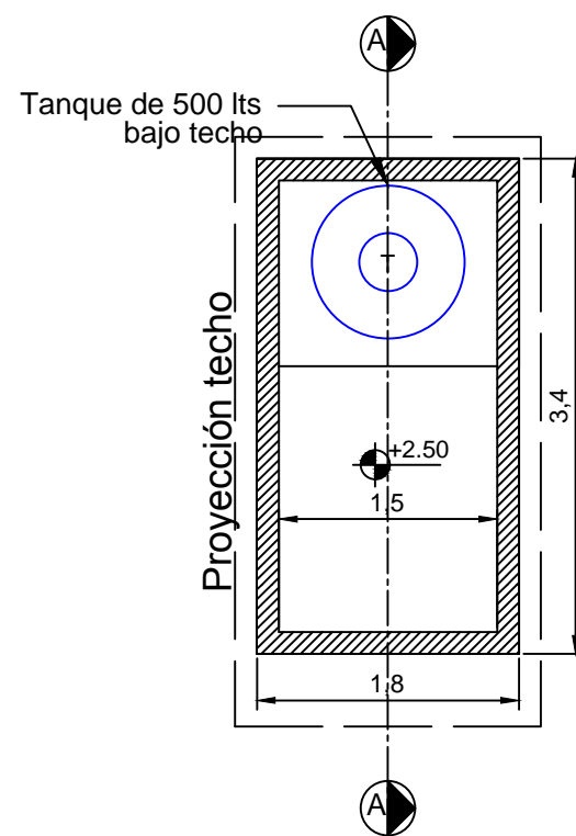
PLANTA +2.50
