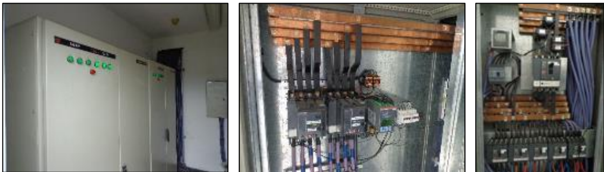
Fotografías TGBT-2 (Sistemas - Data Center). Detalle exterior e interior.
