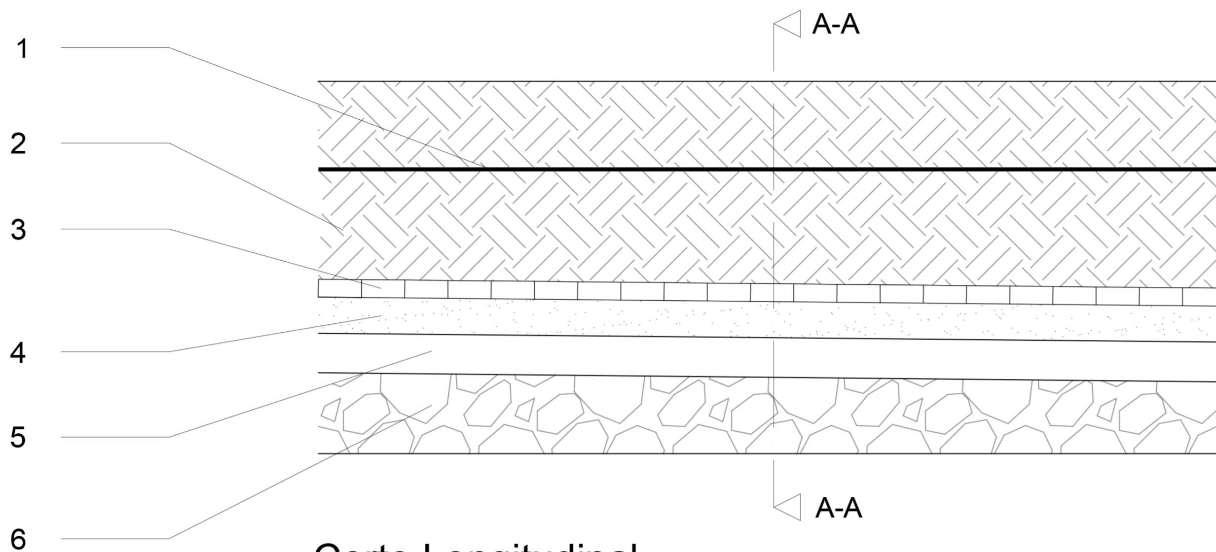
Corte Longitudinal
