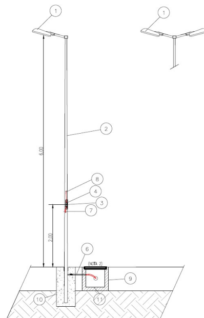
Detalle columna de Iluminación (Ver Anexo III)
