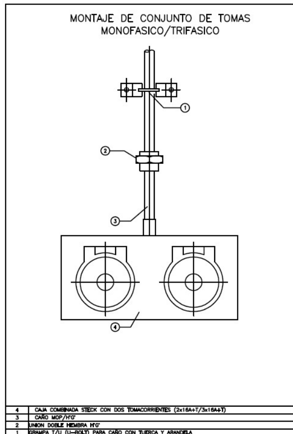
Ilustración de referencia: Montaje de tomas
